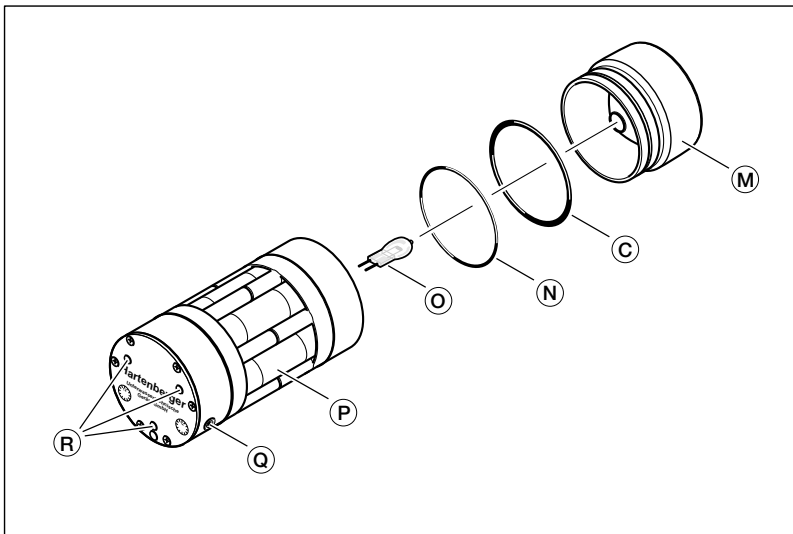
Abb. 2: Gehäuseeinschub
